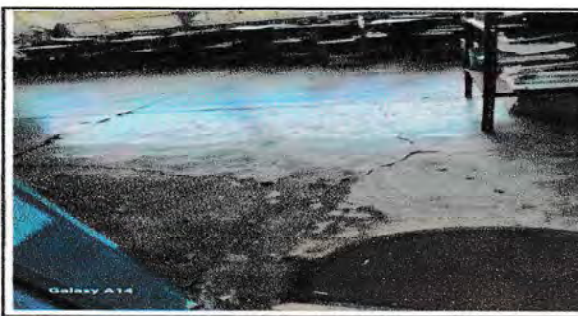
Foto 6: Piso aula No.4 esta aula es la que esta en peores condiciones ya que posee mas grietas y fue lastimada por las raíces de un árbol.
